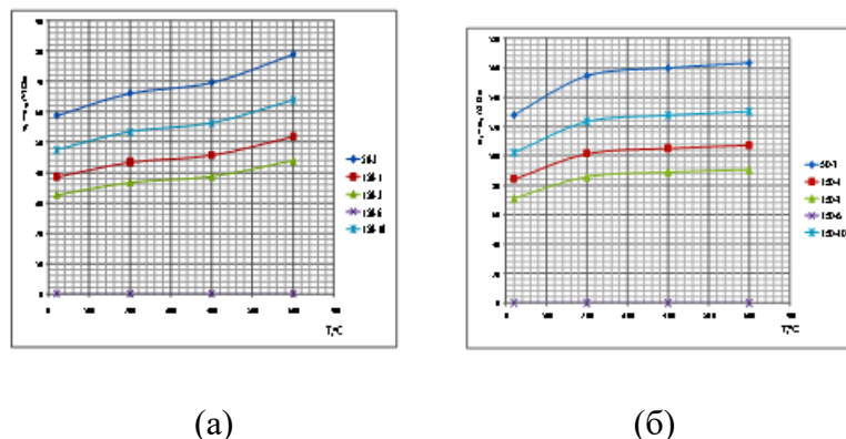
Рис. 1. Зависимость макронапряжений в графите от температуры для параллельных (а) и перпендикулярных (б) слоев при воздействии мощного ионного пучка. Источник: [2]
